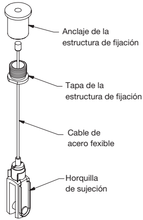
Conjunto del kit de colganteo Blades (Item 6655)
