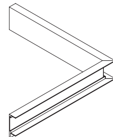
Axiom pour coins intérieurs Interlude
