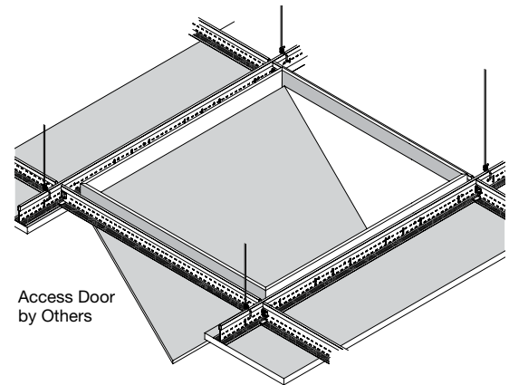
9 Access Door
