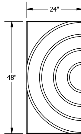
BP6383D45T10-??? RINGS 2X4 TEC DAL FINALE PB PANEL SCALE 1 : 25
