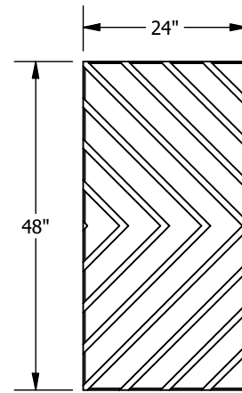
BP6383D42T10-??? TILTS D 2X4 TEC DAL FINALE PB PANEL SCALE 1 : 25
