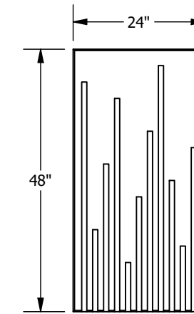
BP6383D54T10-??? LEVELS 2X4 TEC DAL FINALE PB PANEL SCALE 1 : 25
