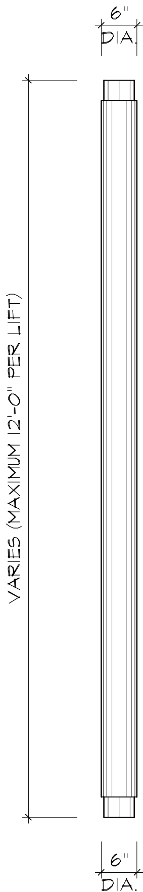
ELEVATION
