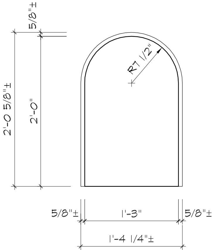
ELEVATION
