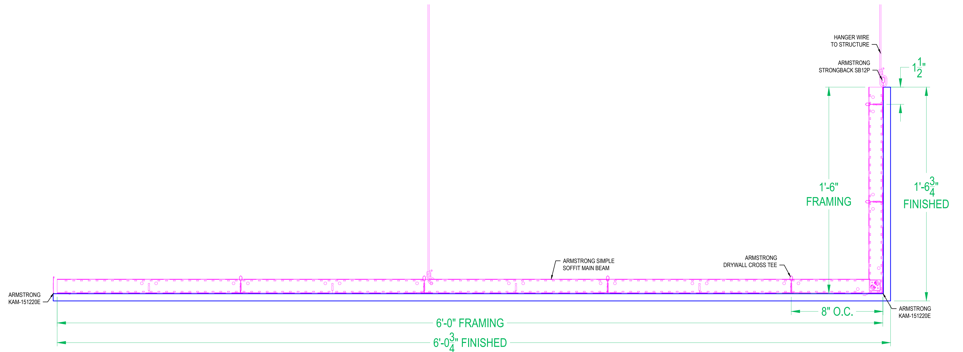
20 SIMPLE SOFFIT SSLU1872
