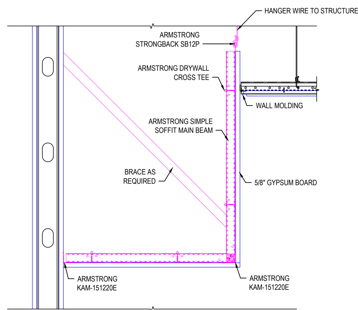
9 SIMPLE SOFFIT L SOFFIT
