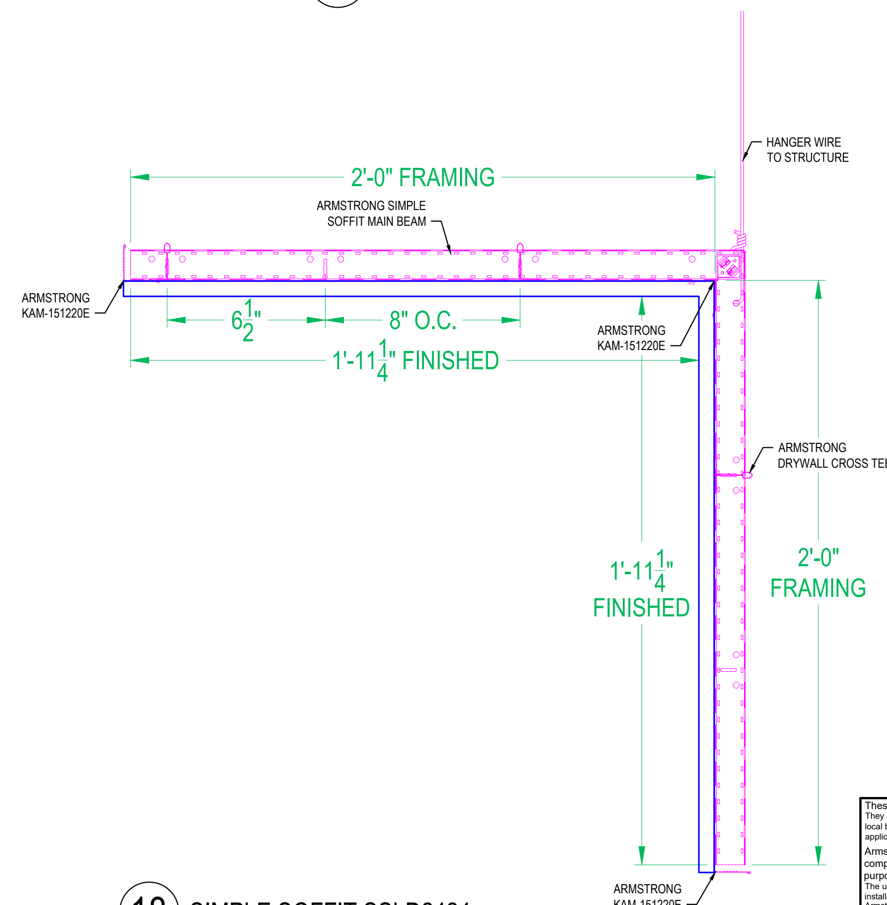
18 SIMPLE SOFFIT SSLD2424
