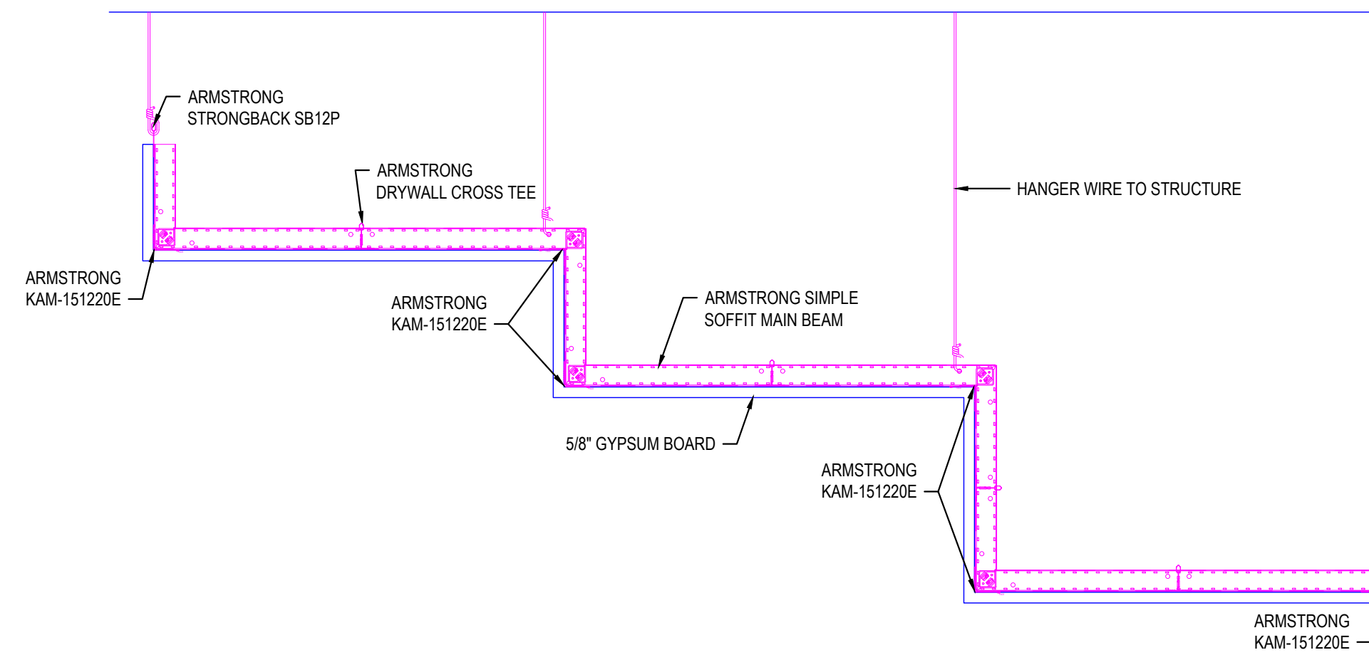
10 SIMPLE SOFFIT STEP SOFFIT
