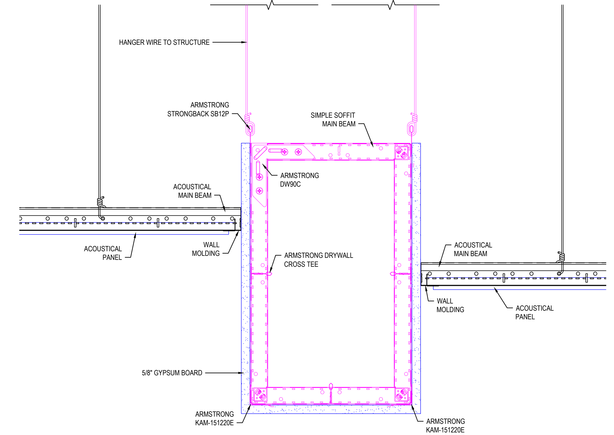
8 SIMPLE SOFFIT SOFFIT BULKHEAD
