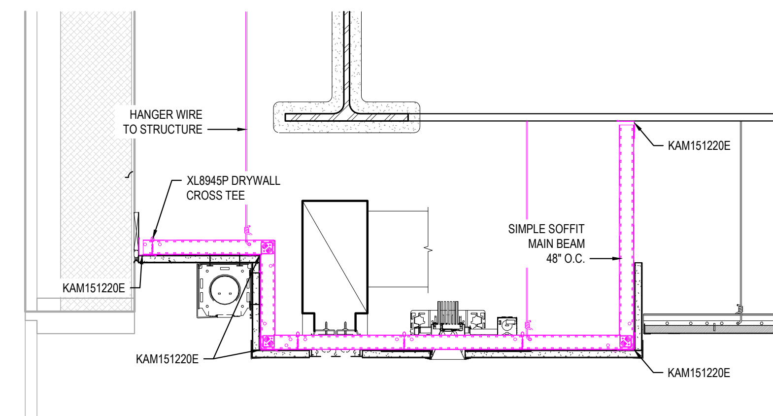
11 SIMPLE SOFFIT CUSTOM SOFFIT
