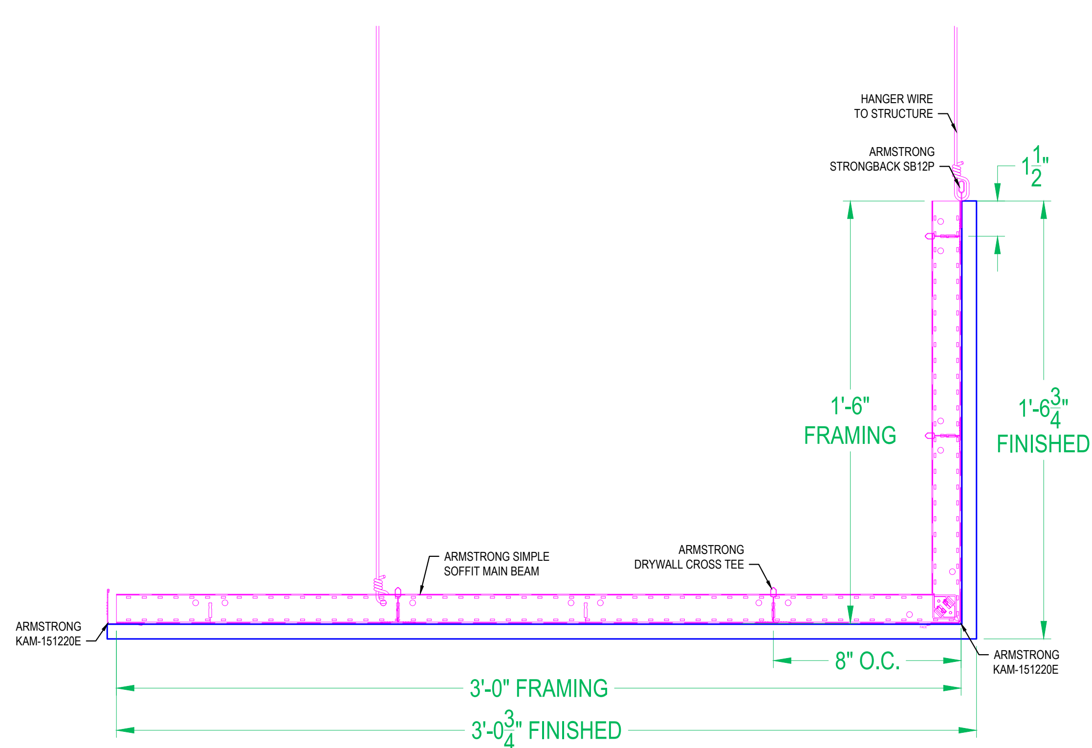
19 SIMPLE SOFFIT SSLU1836
